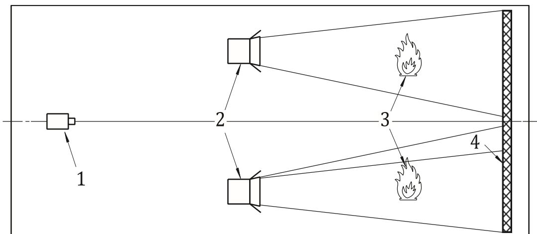
Hình P.2 - Hình chiếu bằng
